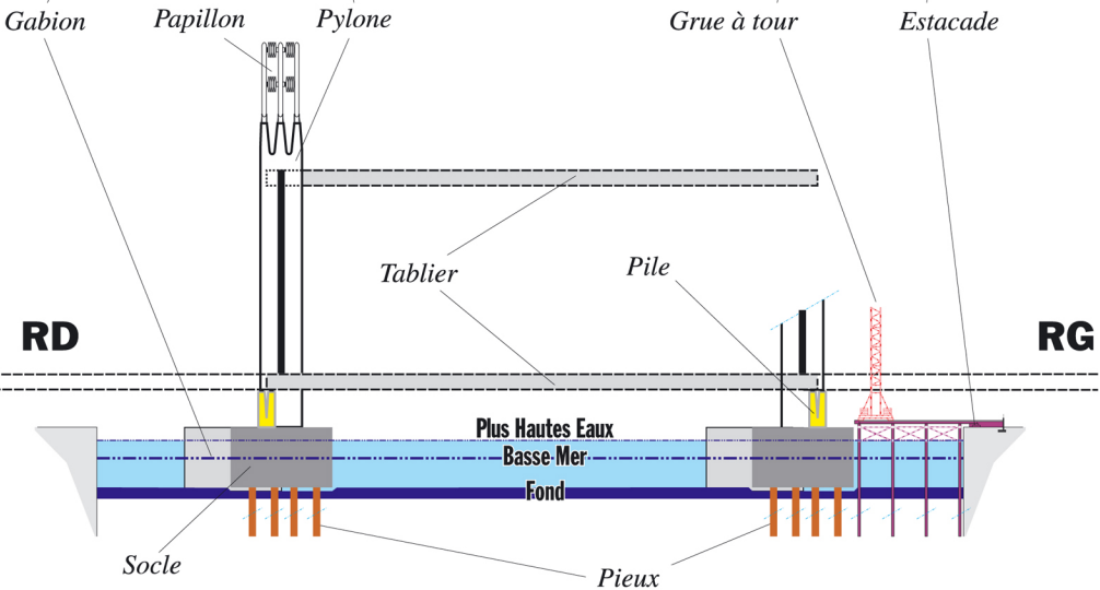
élévation A-A
